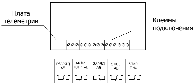
Цоколевка контактов телеметрии и расположение клемм подключения
